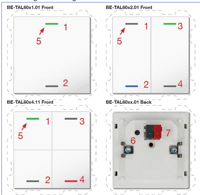
Abbildung 2: Aufbau & Bedienung
